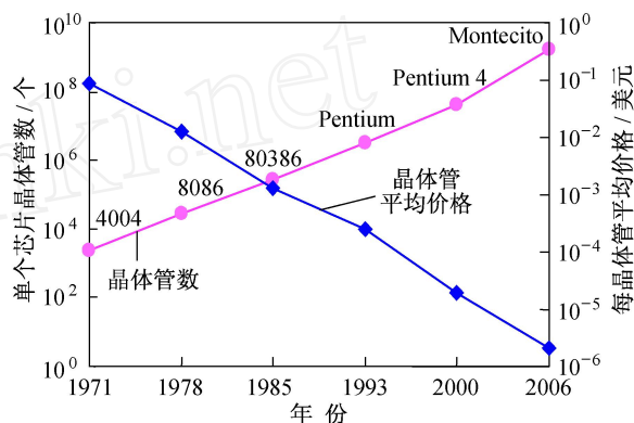
图2 CPU集成度及其所对应的单个晶体管价格
