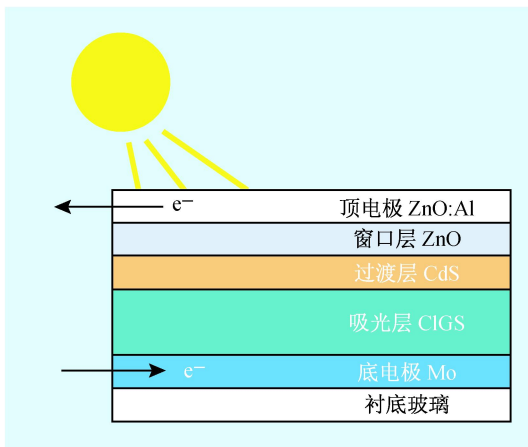
铜铟镓硒[Cu(In, Ga)Se 2 ,简称 CIGS]薄膜太阳能电池主要由底电极、P-N 结 CIGS/ CdS 和顶电极三部分组成;太阳光透过透明导电的 ZnO: Al 层和 CdS 层,辐照到吸光层 CIGS 上激发出额外的电子-空穴对;在 P-N 结电场的作用下,额外产生的电子通过顶电极 ZnO: Al 层输往外电路,空穴则通过底电极 Mo 输往外电路,从而实现了光电转换
