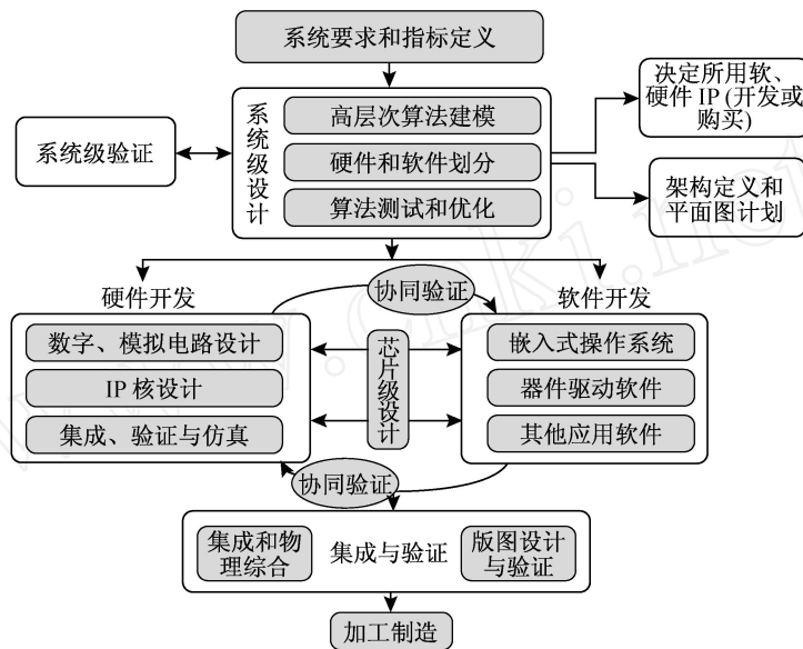
图 13 系统级芯片 (SoC) 简化设计流程
